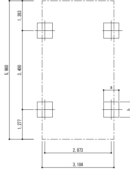
■基礎配置図
